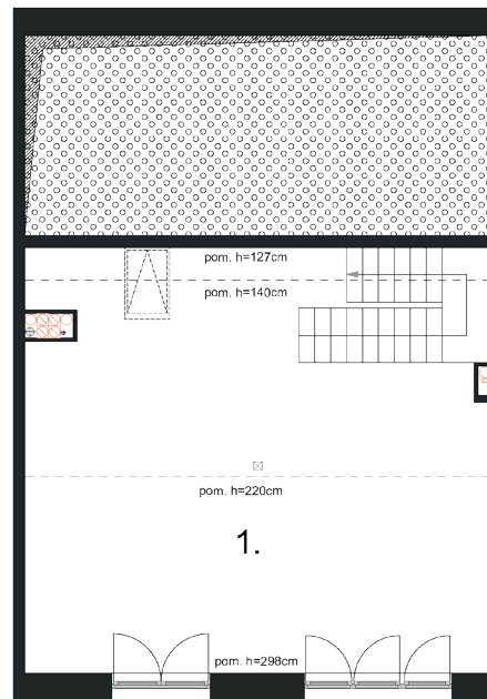
PODDASZE
