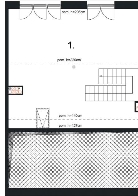
PODDASZE
